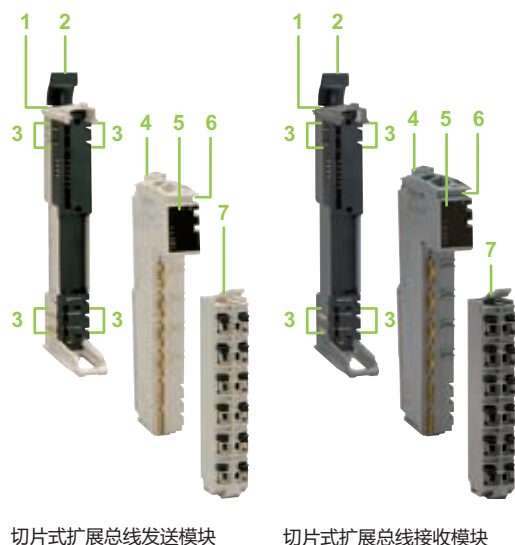
切片式扩展总线发送模块
