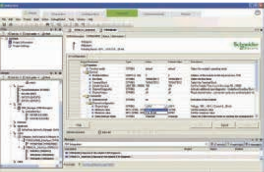
设置切片式模拟量输入扩展模块的参数(IP 20站)
